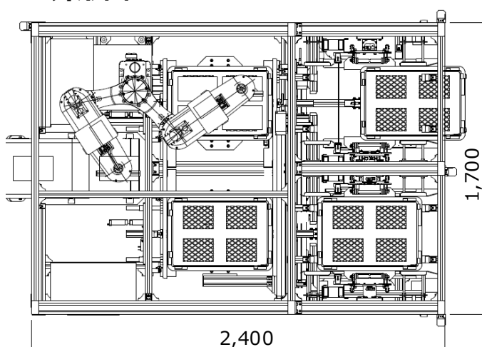
■ 外形図
